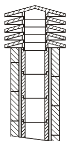
(1) Pot de cheminée industriel à éléments préfabriqués, permet une excellente évacuation des fumées.
